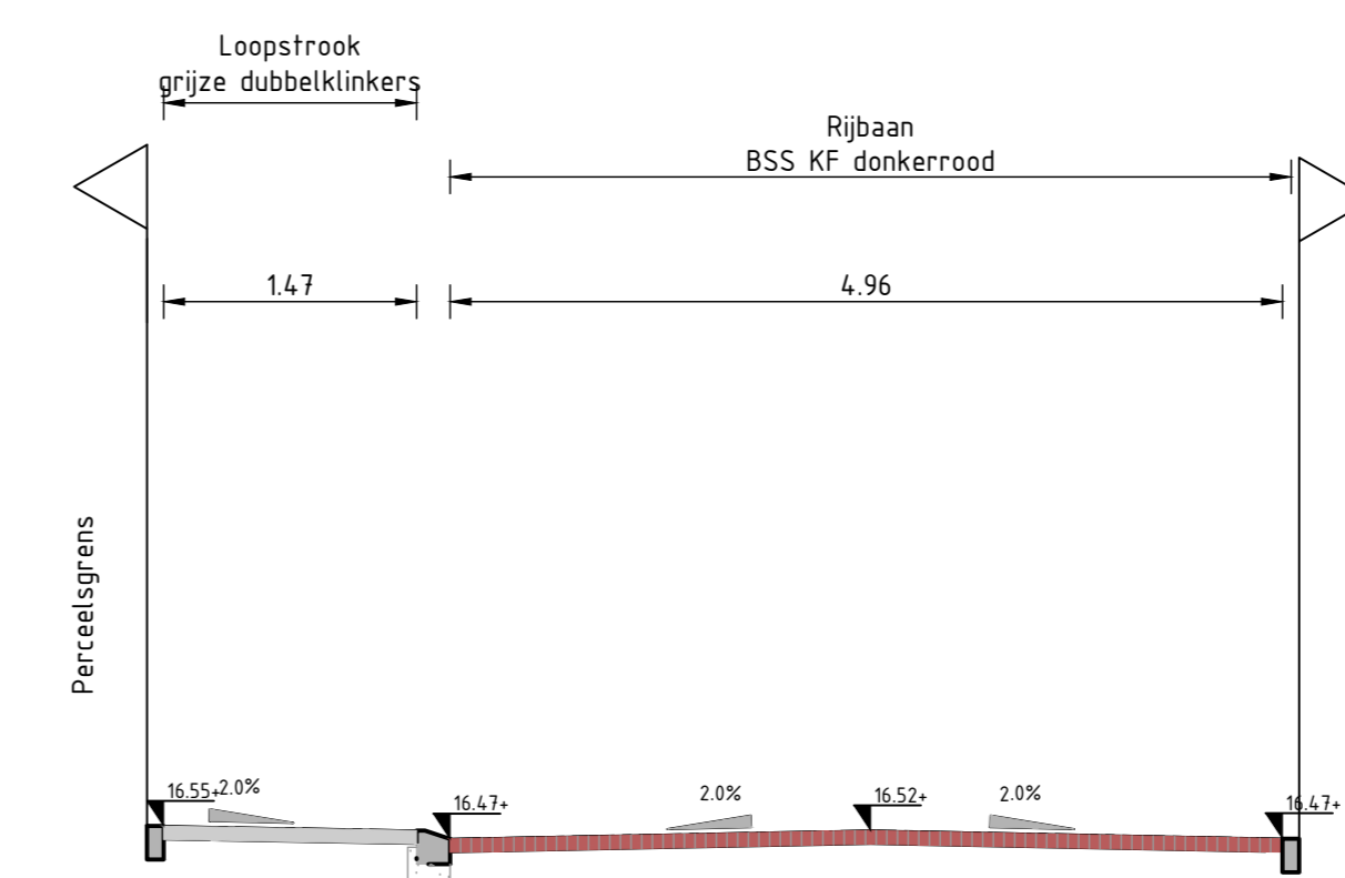
Dwarsprofiel B-B Schaal 1:50
